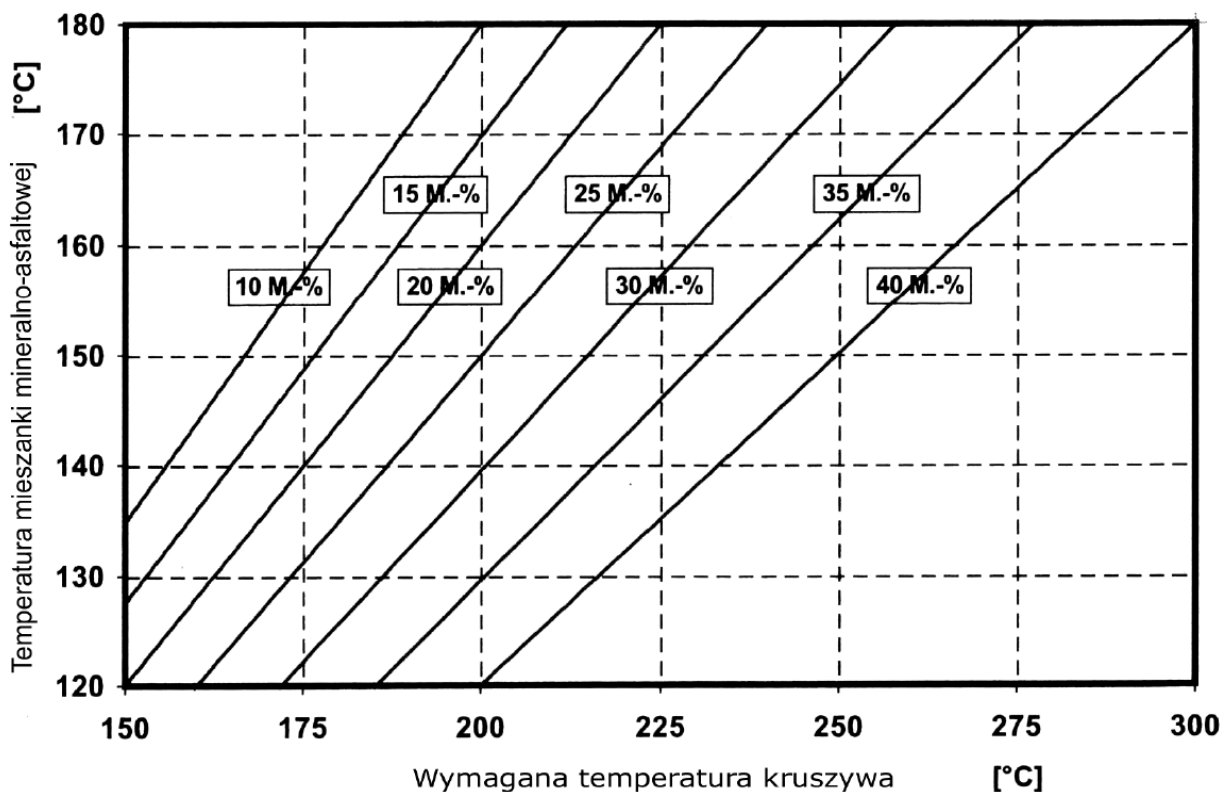
Tablica 8a. Temperatura kruszywa w zależności od ilości zimnego i suchego granulaku asfaltowego
